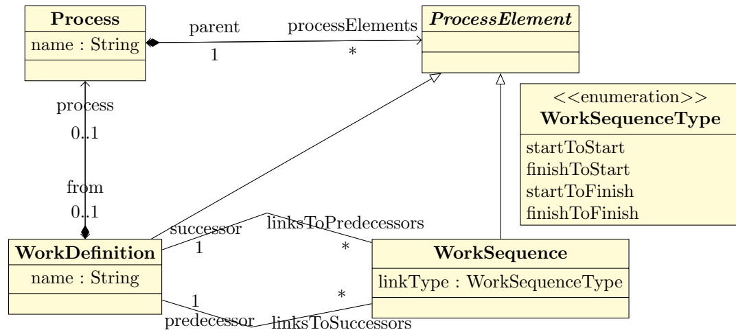
FIGURE 7.1 – Métamodèle SimplePDL.
