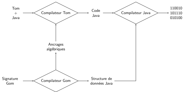
Figure : Processus de compilation d'un programme Tom
